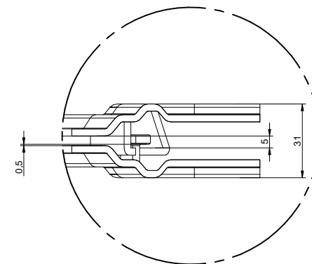
DETTAGLIO C
